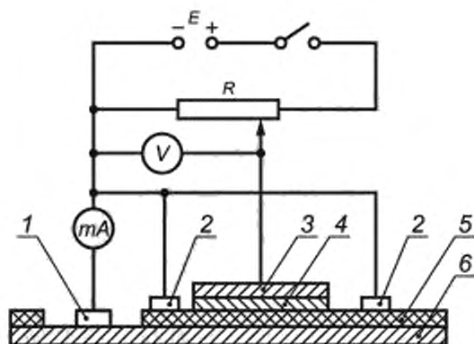
1 — контакт с трубой; 2 — экранирующие кольцевые электроды-бандажи. 3 — кольцевой электрод-бандаж; 4 — тканевое полотно; 5 — защитное покрытие трубы; 6 — стенка трубы; $E$ — источник постоянного тока; $R$ — потенциометр; $V$ — высокоомный вольтметр, $mA$ — миллиамперметр
