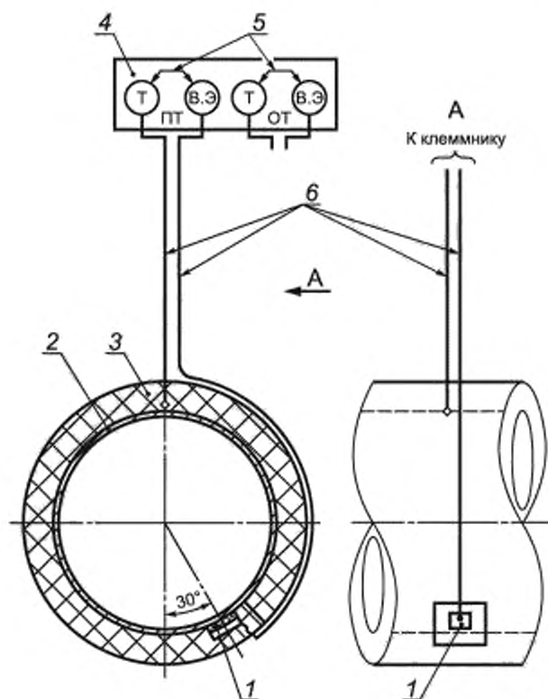
1 — вспомогательный электрод; 2 — трубопровод; 3 — изоляционная конструкция; 4 — клеммная панель контрольно-измерительного пункта для присоединения контрольных проводников от подающего (ПТ) и обратного (ОТ) трубопроводов; 5 — электрическая перемычка; 6 — контрольные проводники
