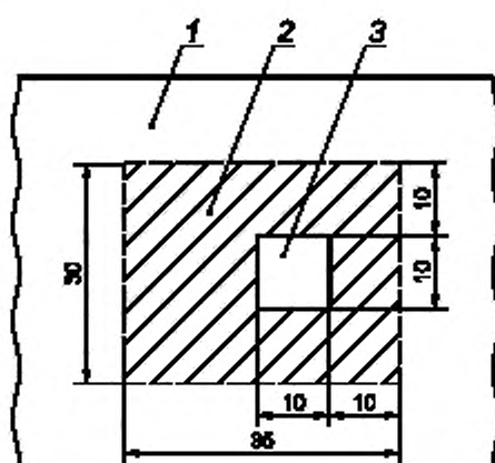
1 — испытуемое защитное покрытие. 2 — расчищенная площадка; 3 — образец покрытия для сдвига
