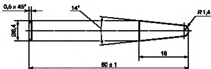
Рисунок Ф.2 — Размеры резца для выполнения прорезания
